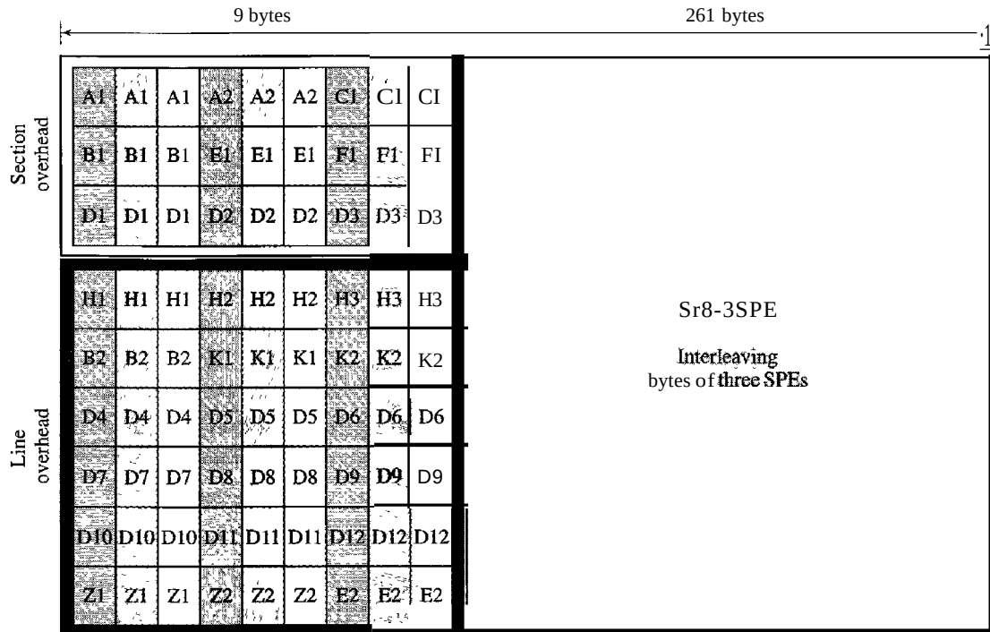
Figure 17.14 AnSTS-3frame
